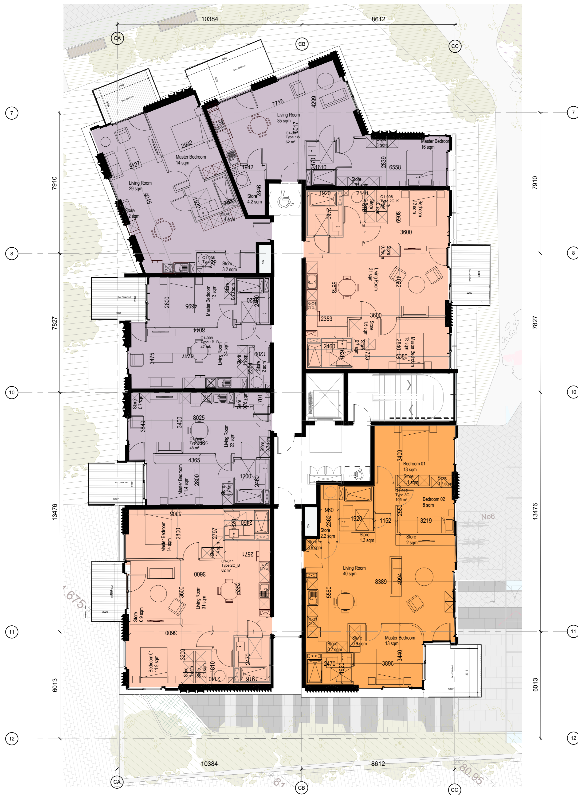
1 01 FFL GA Part V Block C 1 : 100
